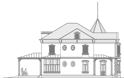
Elevação 03
