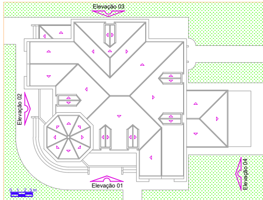
Implantação e Cobertura
