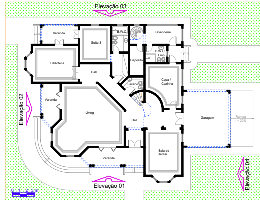
Térreo
